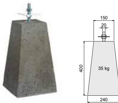
Betonpoer verstelbaar
