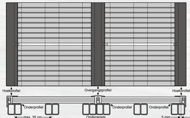
Detailtekening:
