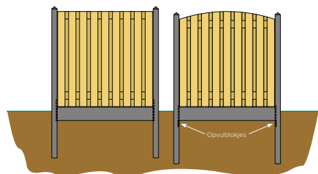
Montage voorbeeld
