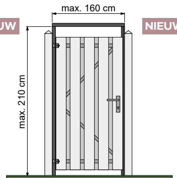
Universeel tuindeurkozijn
